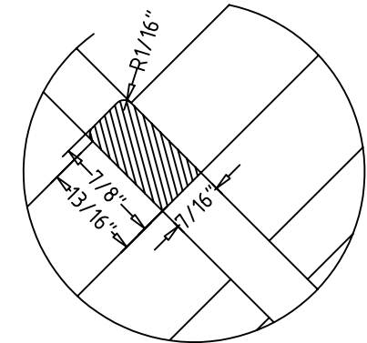
Detail A-A
