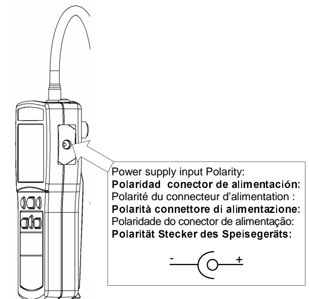
Fig. 3: Power supply input / Conector alimentación / Connecteur d'alimentation / Connettore alimentazione / Conector de alimentação Abb. 3: Der Stecker des Speisegeräts
