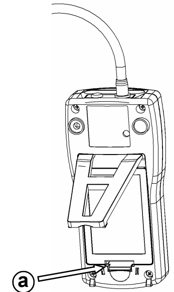
Fig. 2: Battery compartment / Acceso compartimento pilas / Accès au logement des batteries / Accesso vano pile / Accesso ao compartimento das pilhas. Abb. 2: Zugang zum Batteriefach
