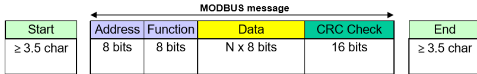
RTU Message Frame
