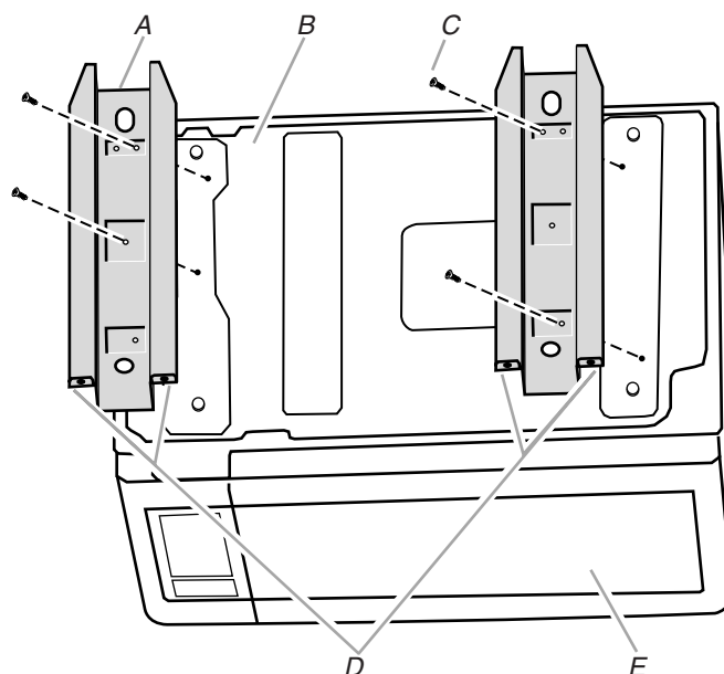
A. Glissières (2) D. Rebords B. Plancher du four à micro-ondes E. Porte C. Vis courtes (4)
