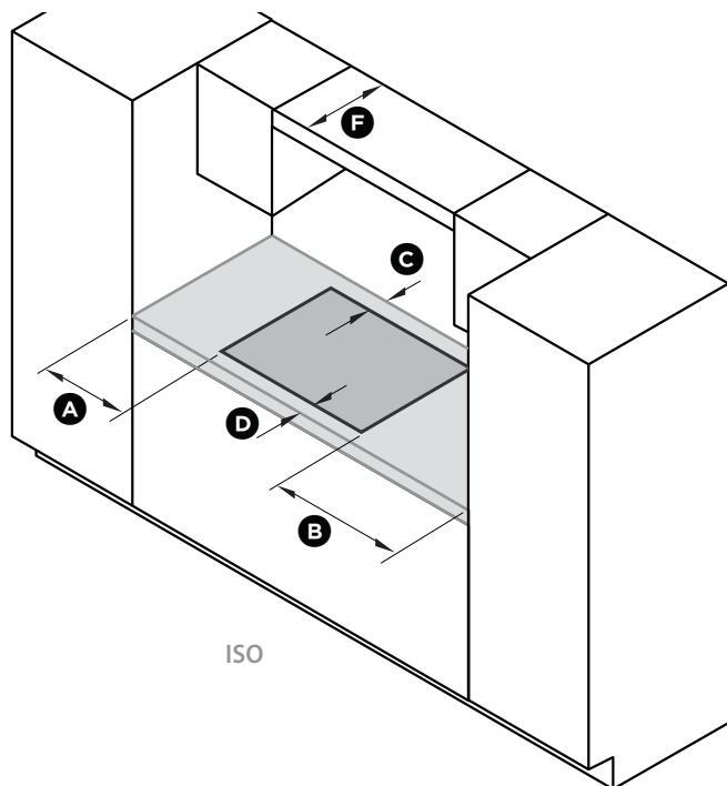
Dimensions de dégagement (mm)
